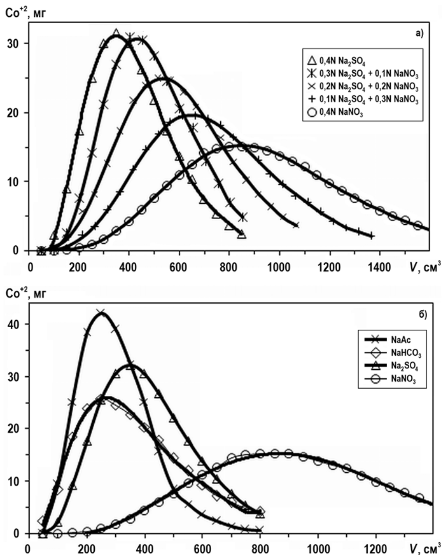
Рис. 2. Выходные кривые элюирования Co^{+2} из сульфокатионита Dowex-50x8 смешанными (а) и индивидуальными (б) солями натрия
