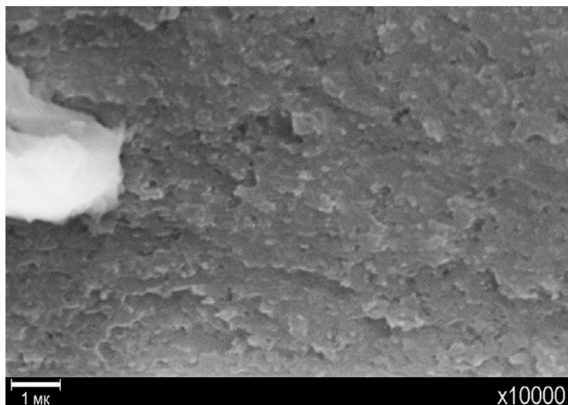
Рис. 2. Горизонтально-слоистая структура многослойного кристалла (аэрогель – 0,01 мас.%)
